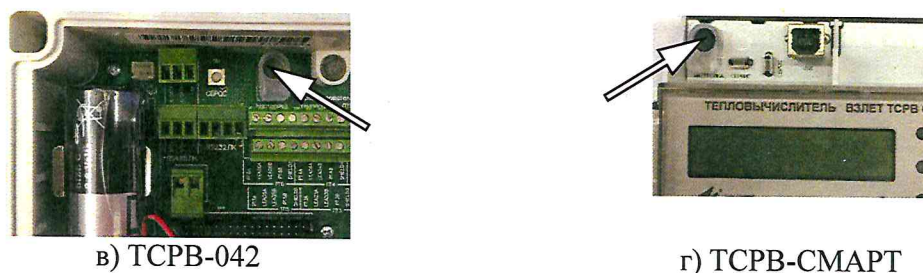
Рисунок 3 – Места пломбировки от несанкционированного доступа тепловычислителей ВЗЛЕТ TCRB
