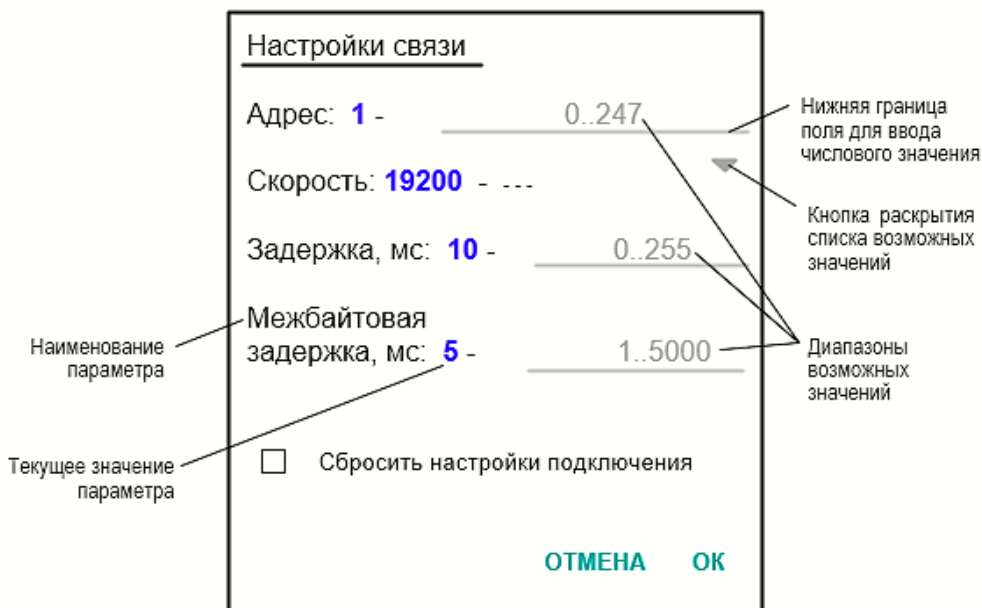
Рис.6. Вид окна редактирования значений установочных параметров.
